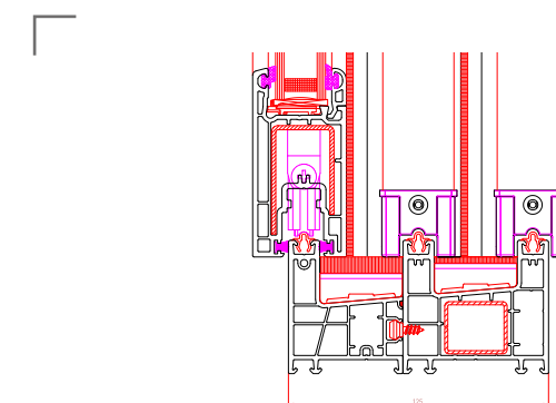
Sección inferior puerta
